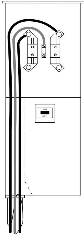
1Ø, CL200, 3W, 120/240V
